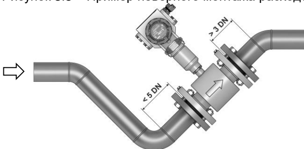
Рисунок 3.6 – Пример возможного монтажа расходомера
