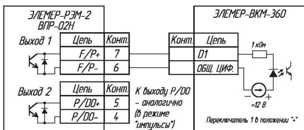
Рисунок А.6 – Схема электрическая подключений вычислителя расхода универсального «ЭЛЕМЕР-ВКМ-360» к дискретным выходам ЭЛЕМЕР-РЭМ-2 с ВПР-02Н. R_H = 1\text{ кОм} . Подключение к цепям «+FP2» и «-FP2» аналогичное
